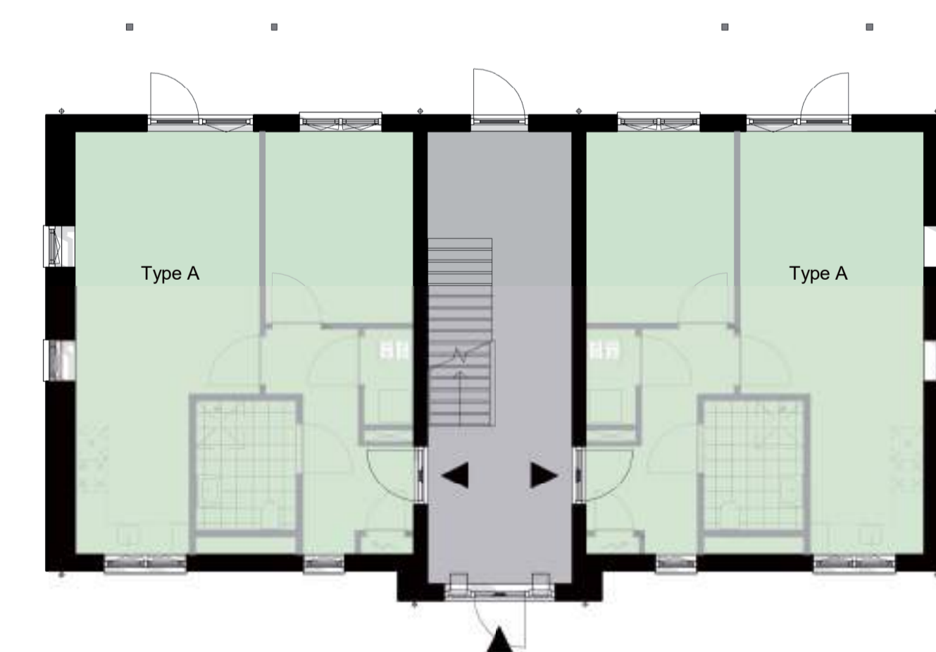
begane grond
