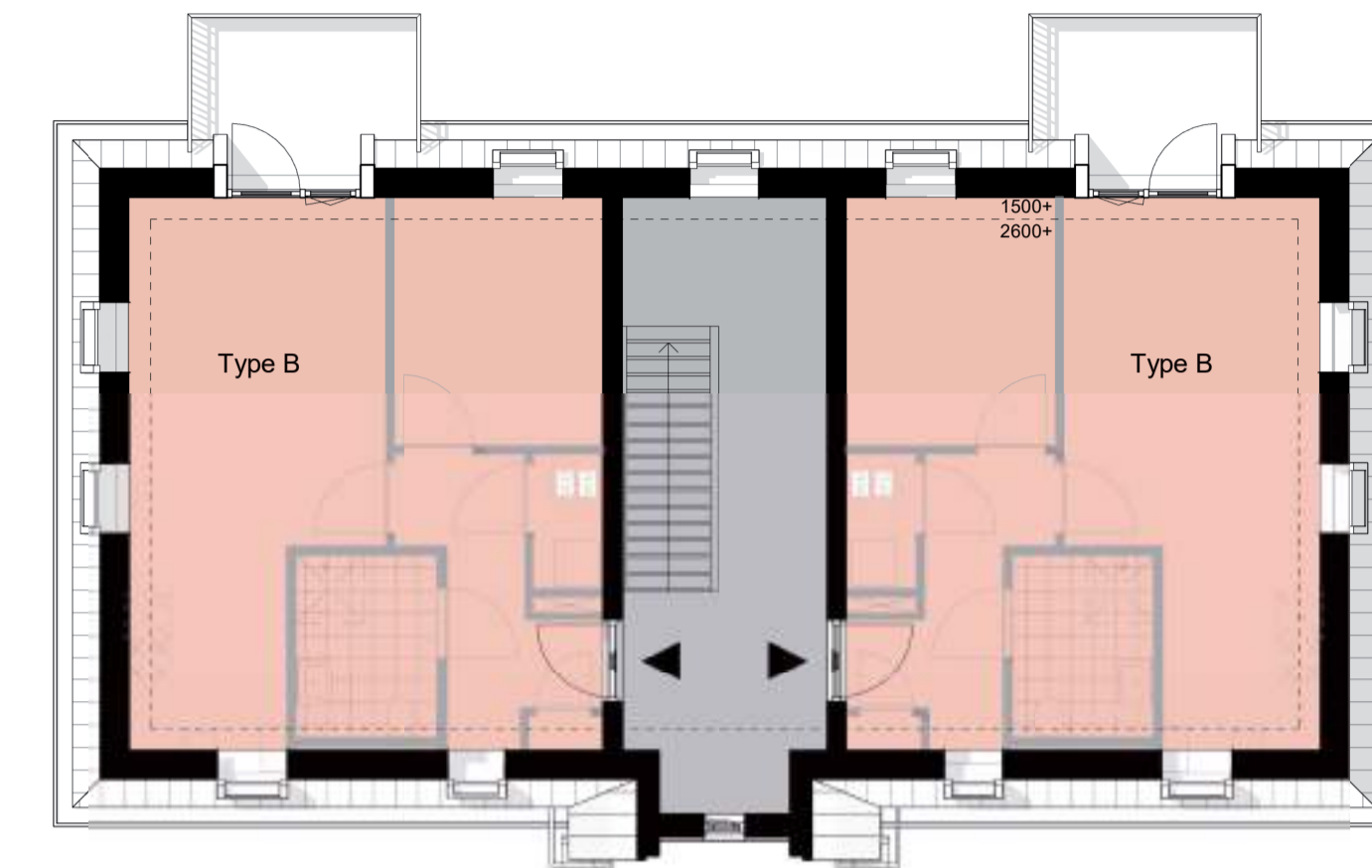
tweede verdieping
