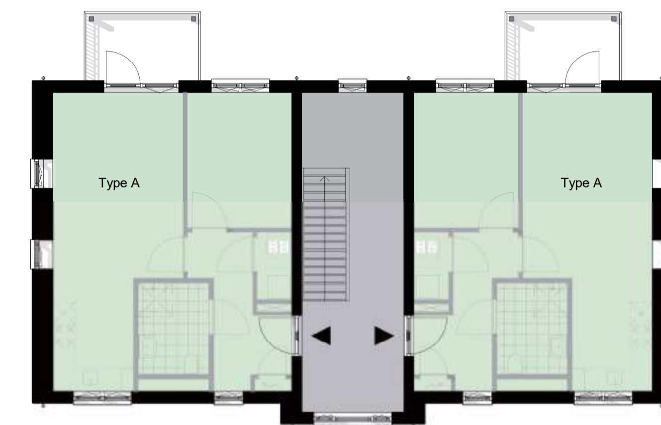
eerste verdieping
